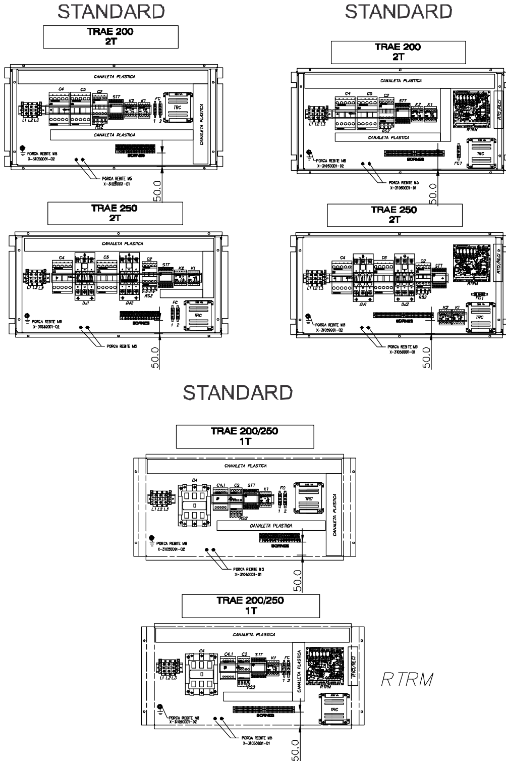
Fig. VII-37 - Layout - TRAE 200/250.
