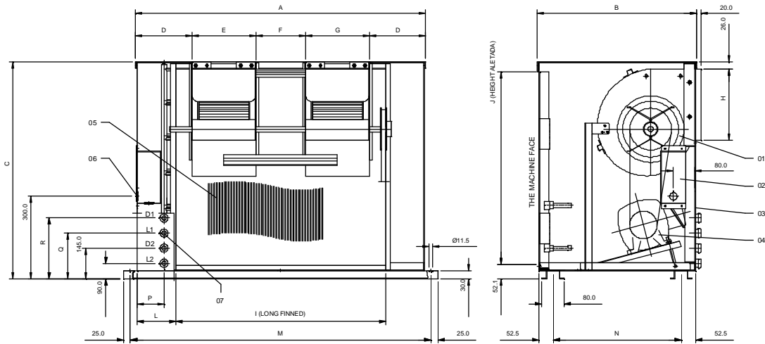
Fig.VIII-14- Dimensions CRCB 050 to 150.
